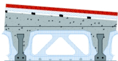
cubierta invertida
